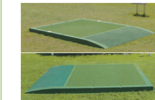
FRPバリアフリースタート台(スロープ型) 商品番号 NTX-SM 003 1700×2343×100mm (人工芝1500×1500mm)
